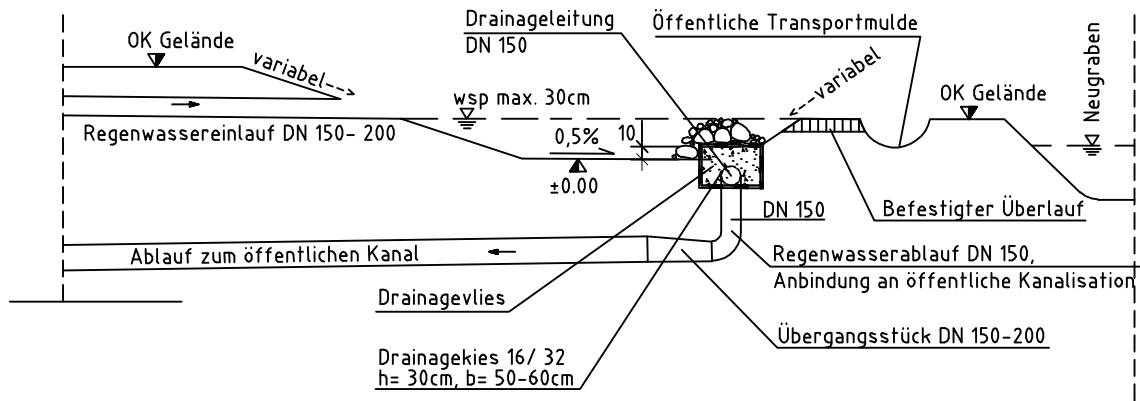
Schnitt
